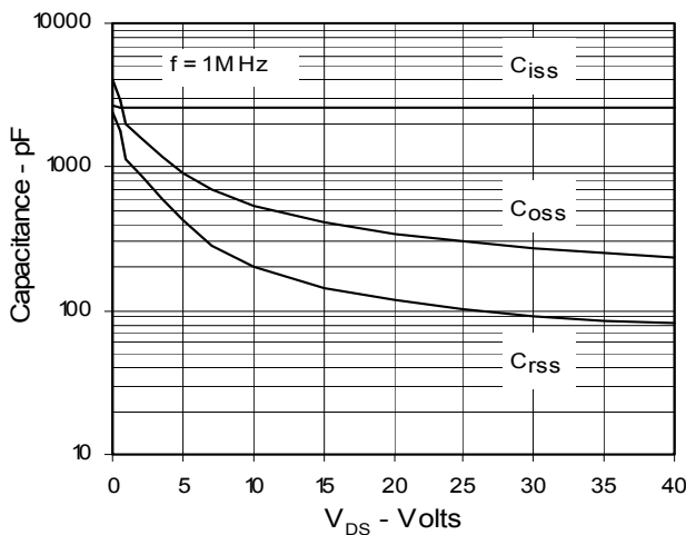
Fig. 11. Capacitance
