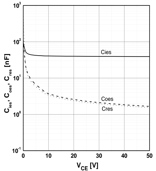
Fig8. Typ. Capacitance
