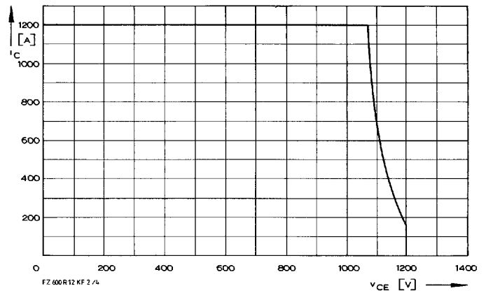
4 Rückwärts-Arbeitsbereich RBSOA. Reverse biased safe operating area. t_{vj} = 125^\circ\text{C} , v_{LH} = 15\text{ V} , R_G = 2\ \Omega
