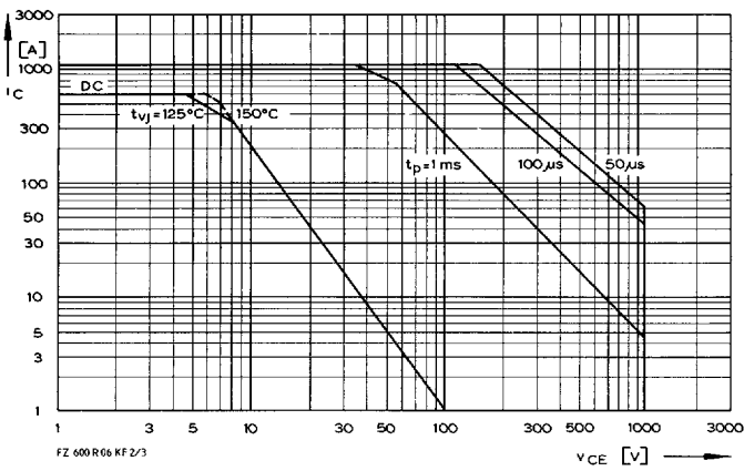
3 Vorwärts-Arbeitsbereich FBSOA (Einzelimpuls, nicht periodisch). Forward biased safe operating area (single pulse, non repetitive). t_{vj} = 25^\circ\text{C}
