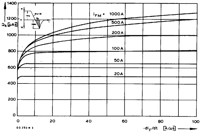
Bild/Fig. 7: Nachlaufladung Q_s in Abhängigkeit von der abkommutierenden Stromstärke -di_F/dt bei t_{vj \max} . Lag charge Q_s versus the rate of decay of the on-state current -di_F/dt at t_{vj \max} .
