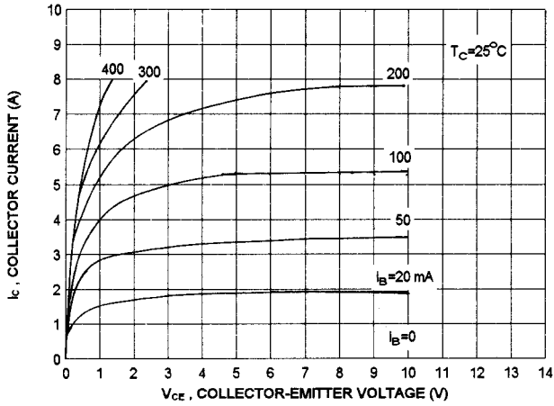
I_c - V_{ce}
