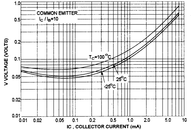
V_{ce(sat)} - I_c
